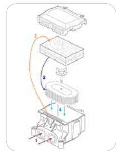
Filtration air
